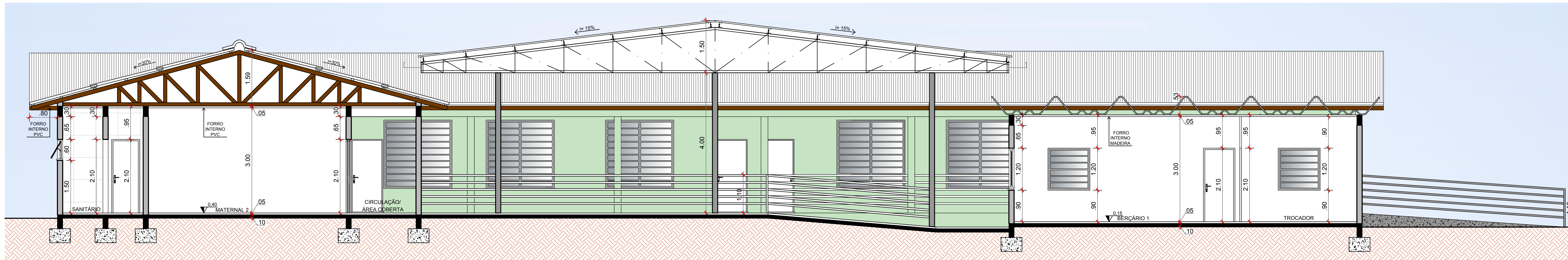
CORTE AA'
